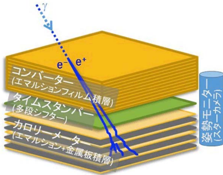
図 1: エマルジョンガンマ線望遠鏡の概念図。エマルジョンフィルムを積層したコンバーター、時刻付与機構多段シフター、姿勢監視スターカメラから構成。コンバーターでガンマ線電子対生成反応を捉え、時刻付与機構で時刻情報を付与し、姿勢監視データと併せることで天球上の到来方向が決定できる。
