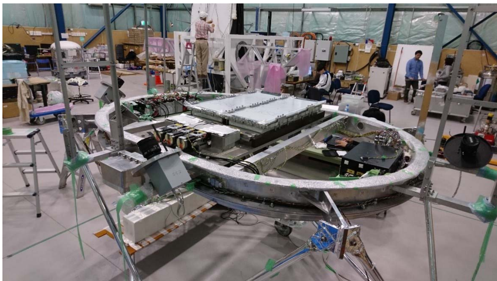
図 2: 気球実験最終準備時の様子。与圧容器リング内側(短手方向 1.5m)に多段シフターを搭載し、その上にエマルジョンフィルムパックを搭載している。エマルジョンフィルムは 1 ユニットあたりの大きさが 37.8cm×25cm、厚み方向に 113 枚積んでいる。それらを 4 ユニット並べ、口径面積 3780cm 2 を実現している。与圧容器リング外側には 3 方位を向いたスターカメラのレンズ(黒)が見える。
